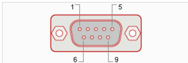
D-Sub 핀 배정
